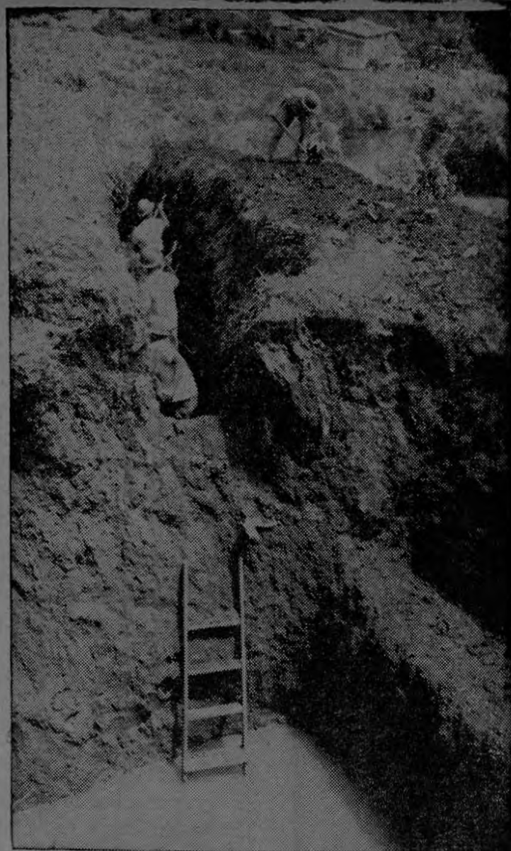
TRABAJOS DE ALCANTARILLADO REALIZA EL SNA. Pueden verse en esta fotografía los trabajos que está ejecutando el Servicio Nacional de Acueductos y Alcantarillado en el Barrio Betania y que consisten en una excavación para instalar un tanque séptico, en primer plano, y en el drenaje del mismo hacia el Río Torres. El SNA instaló también, en el Barrio Córdoba, una tubería de aguas negras de 600 metros de longitud, hasta el colector del sur, en el Río Ocloro y otra línea de alcantarillado de los edificios del Poder Judicial a la avenida 12. Estas obras constituyen un adelanto del magno proyecto de alcantarillado sanitario para el área metropolitana de San José, que se construirá con el préstamo del BID para el programa de las cinco ciudades.
